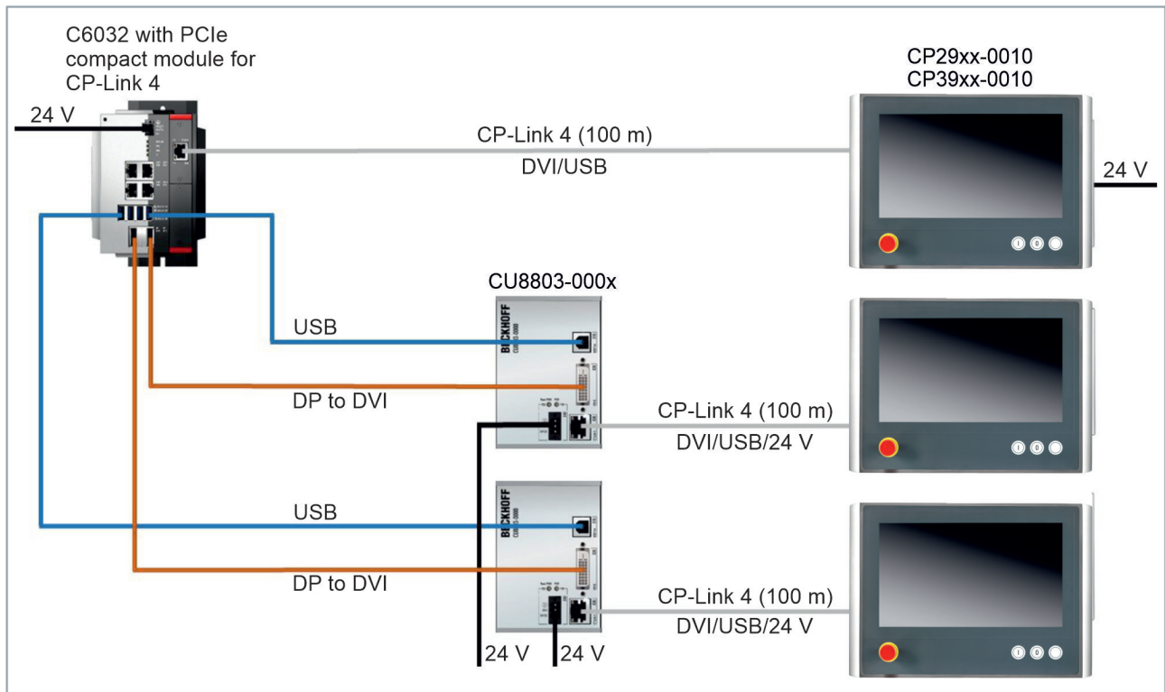
Fig. 14: CP-Link 4, CU8803
