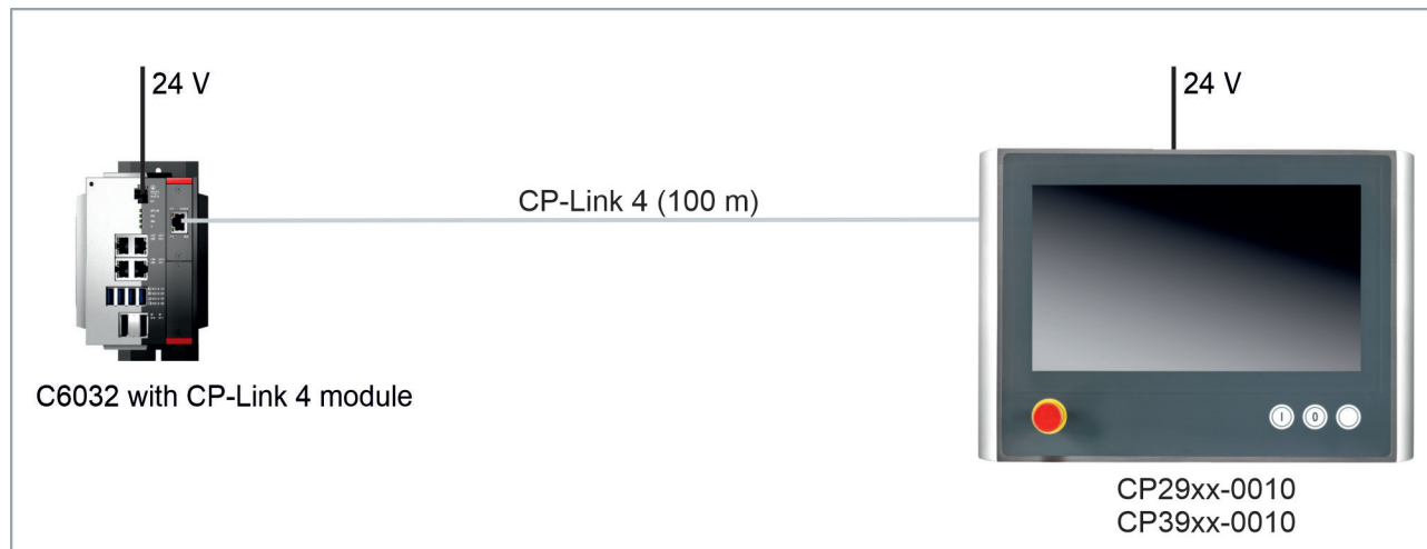
Fig. 12: CP-Link 4
