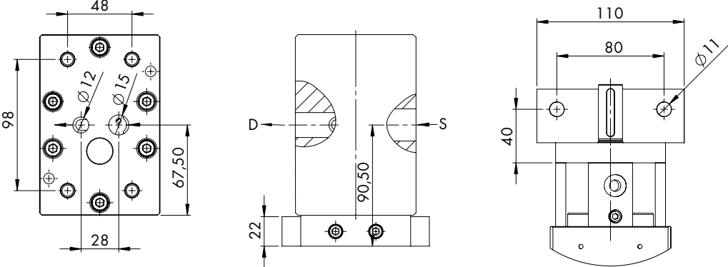
Ansicht/View A - mit Pumpenfuß und Anschlussplatte/ with foot bracket and connection plate
