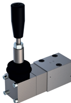
Manual actuation
